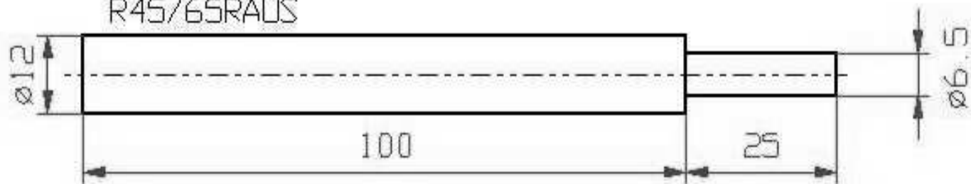
R45/65REIN
