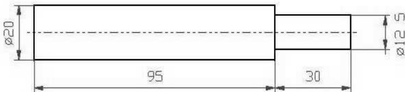
Kolbenbolzenaustrreiber
