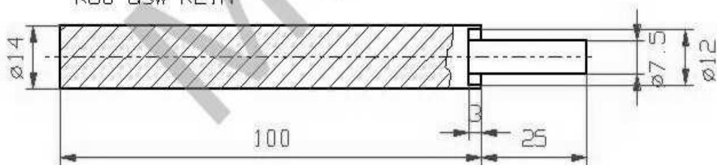
Kolbenbolzenaustrreiber
